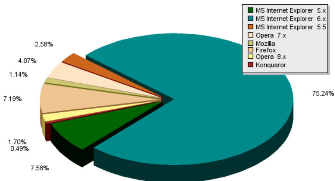
Диаграмма 6. Броузеры
